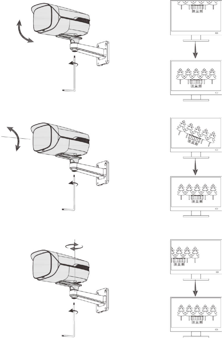
图3-9 调节角度
