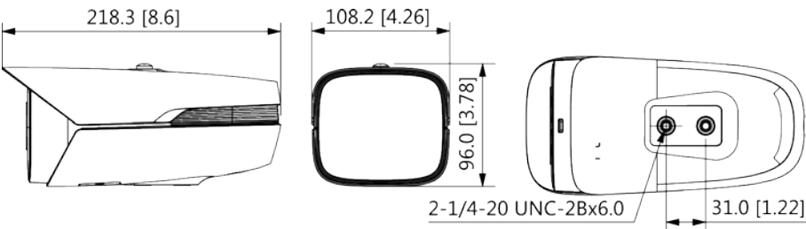
图3-2 结构尺寸
