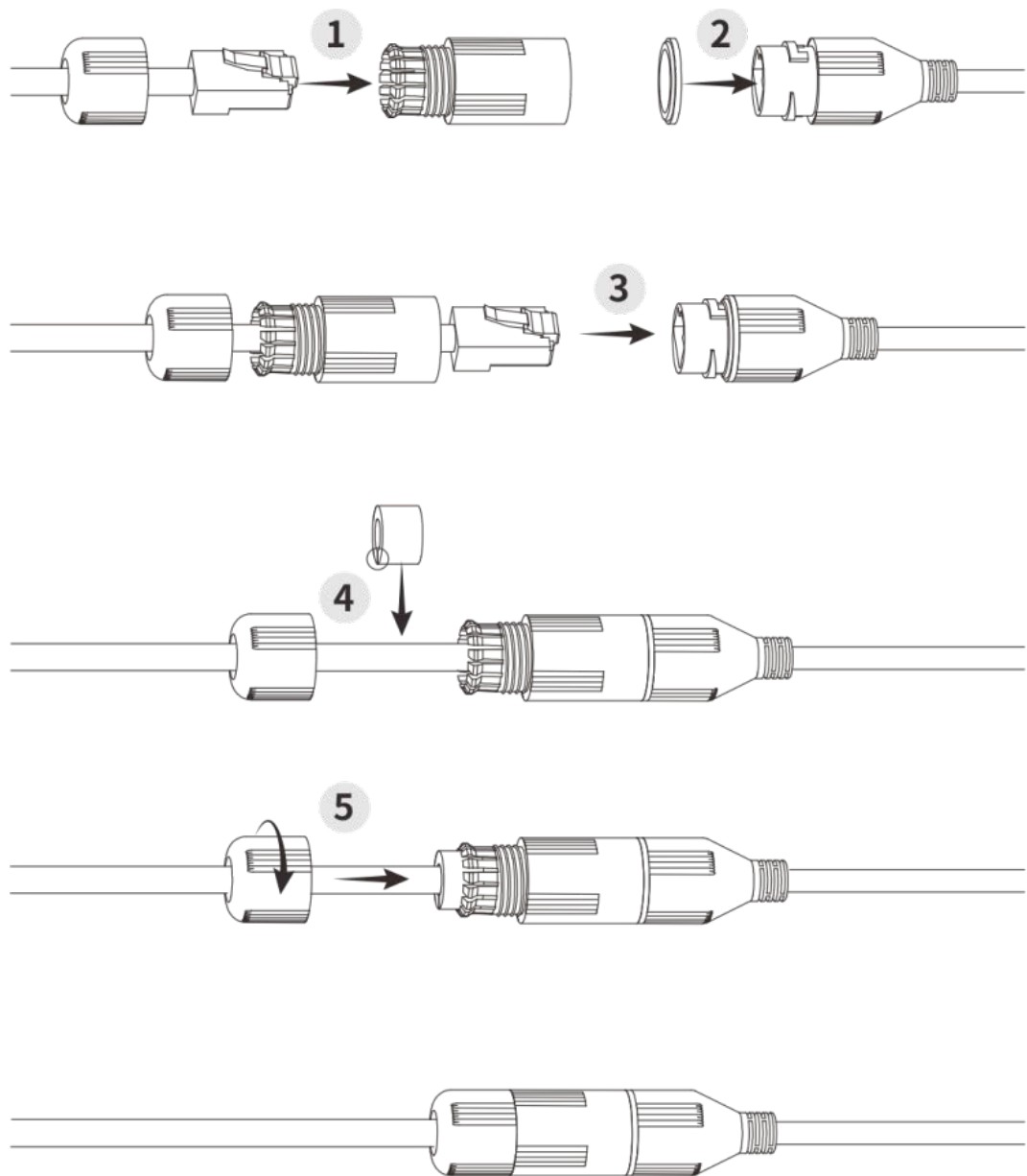
图3-8 安装网口防水套
