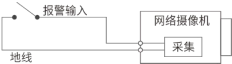
图1-2 报警输入
