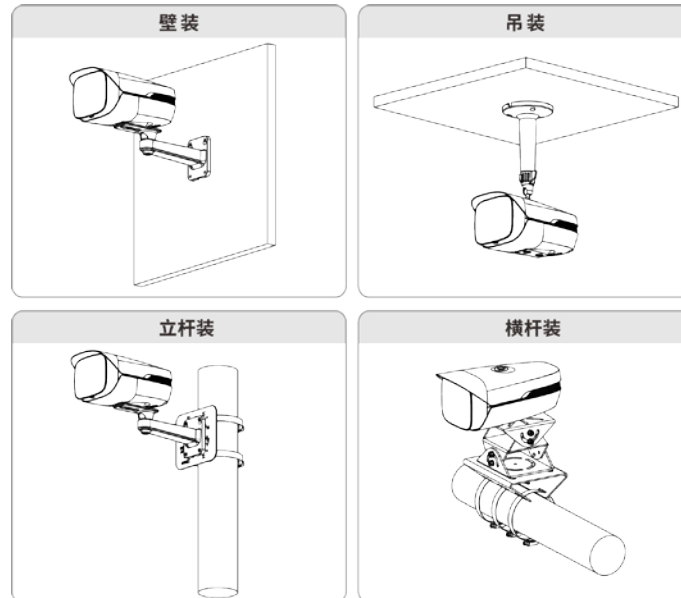
图3-4 安装场景
