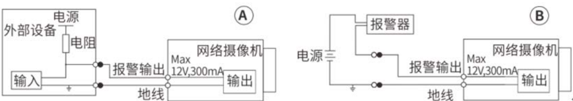
图1-3 报警输出
